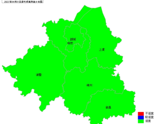
2023年04月01日累计春茶采摘适宜率图
