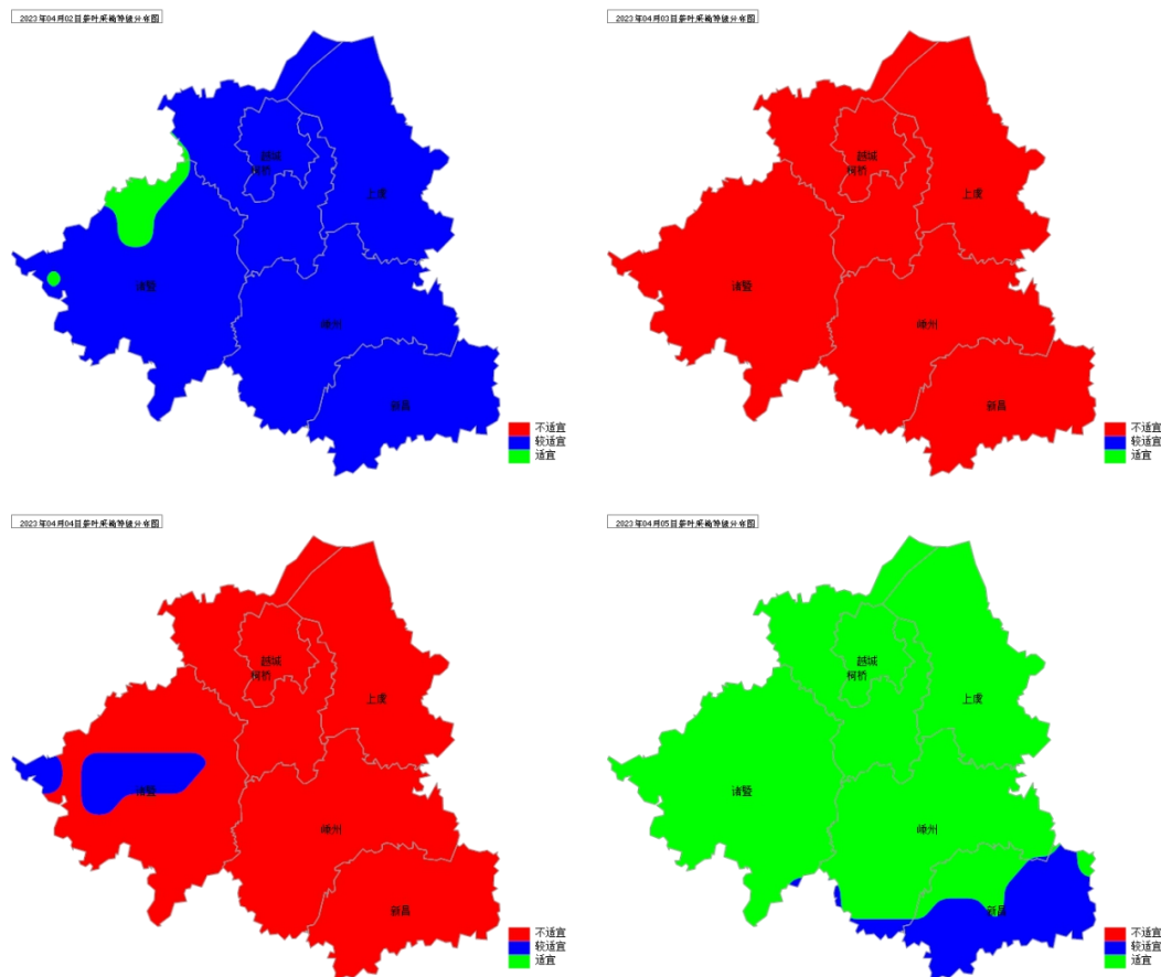
图1 3月27日-4月5日绍兴市春季采摘适宜度指数
