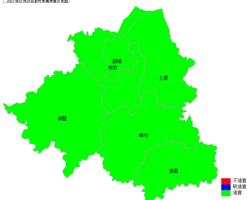
2023年03月30日累计春茶采摘适宜率图
